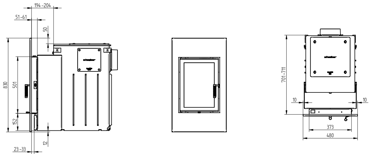
Door frame 37/50 90 mm thick. 5 mm
