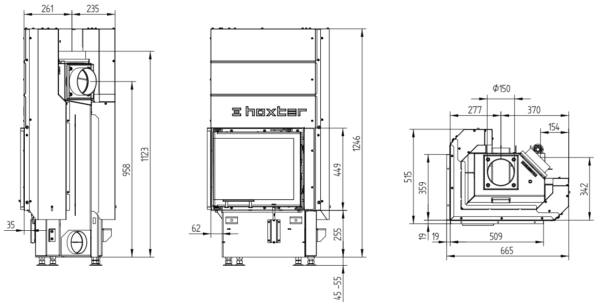
ECKA 50/35/45Lh left liftdoor
