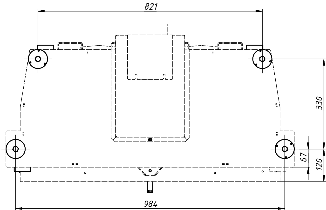
Розташування ніжок (вид знизу)
